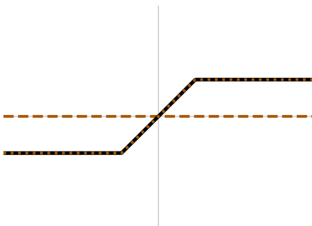
Hard tanh
