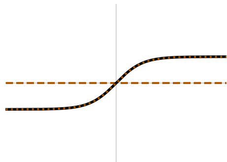
tanh
