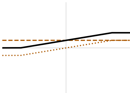
Hard sigmoid
