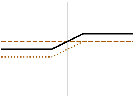
Sparse sigmoid
