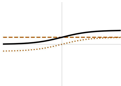
Sigmoid
