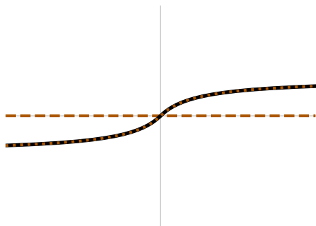
Softsign
