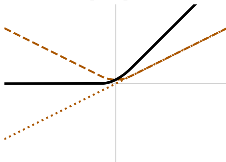
Sparseplus
