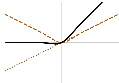
GELU
