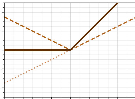
sparse_plus
