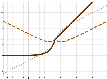
selu
