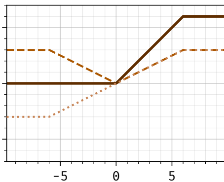
relu6
