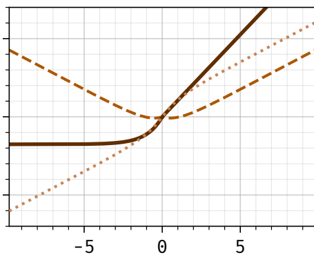
selu
