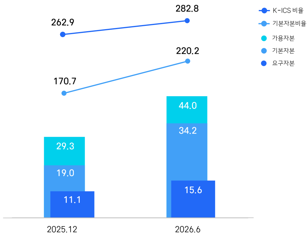
K-ICS 비율 (% , 조원)
