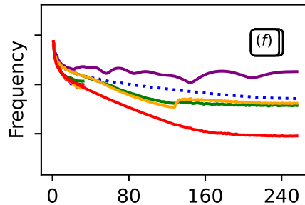
Test Res. 512*
