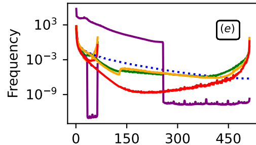
Test Res. 1024
