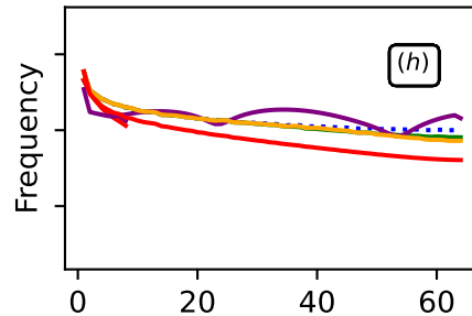
Test Res. 128
