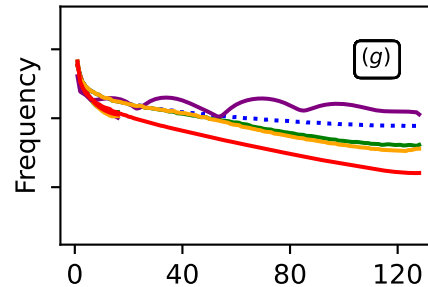
Test Res. 256
