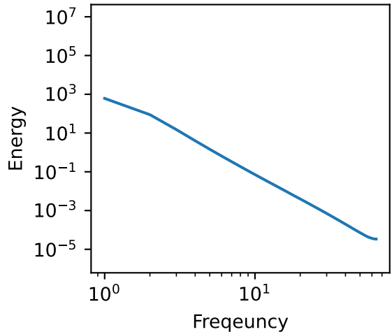
Darcy (2D)
