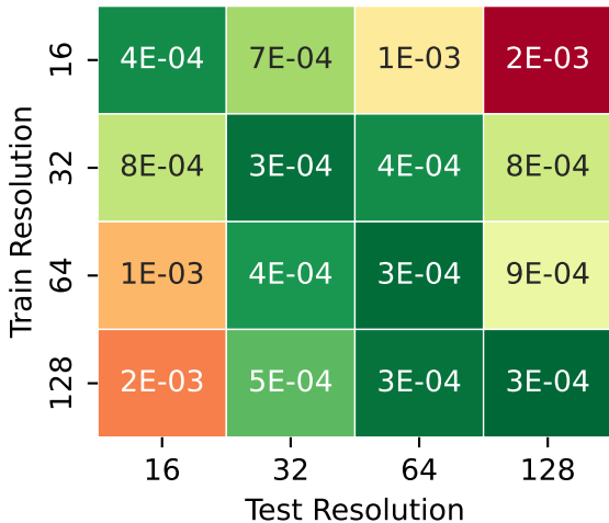
GeLu
