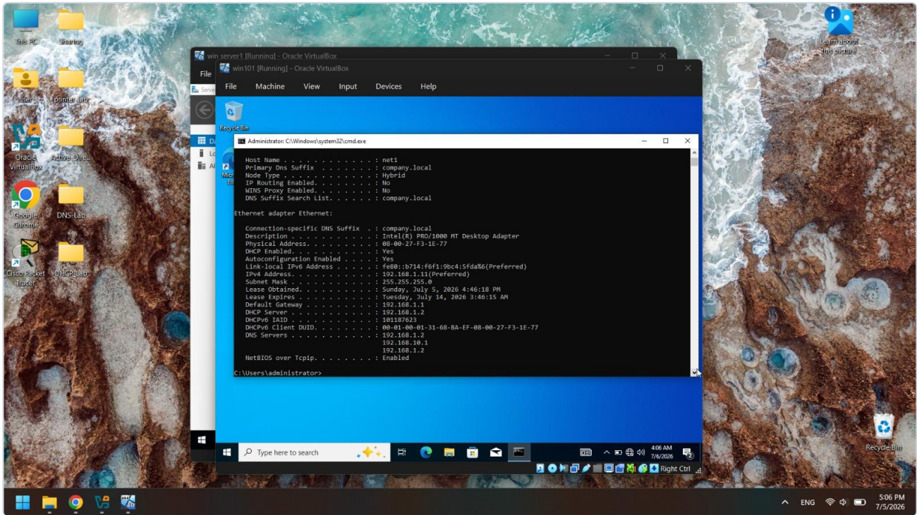
Şəkil 3: Net1 müştəri maşınının IP konfigurasiya məlumatları
