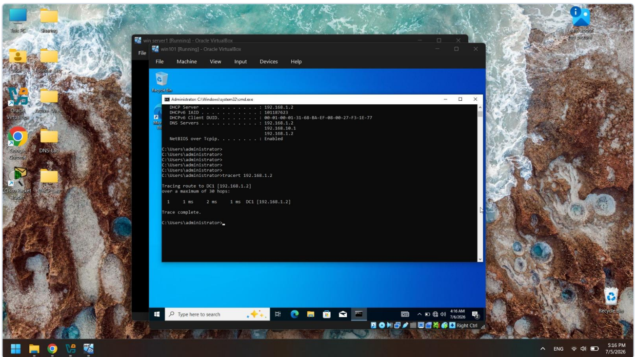
Şəkil 5: Net1 maşınından serverə doğru marşrutun (tracert) izlənilməsi
