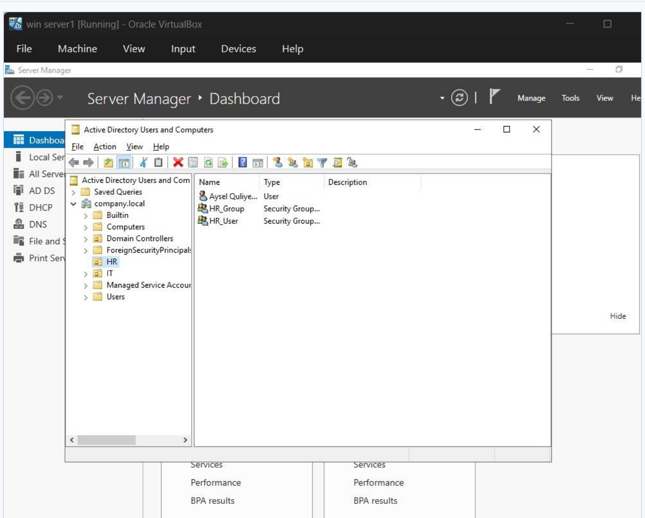
Şəkil 3: HR Organizational Unit (OU) strukturu, qrupları və istifadəçi hesabı.
