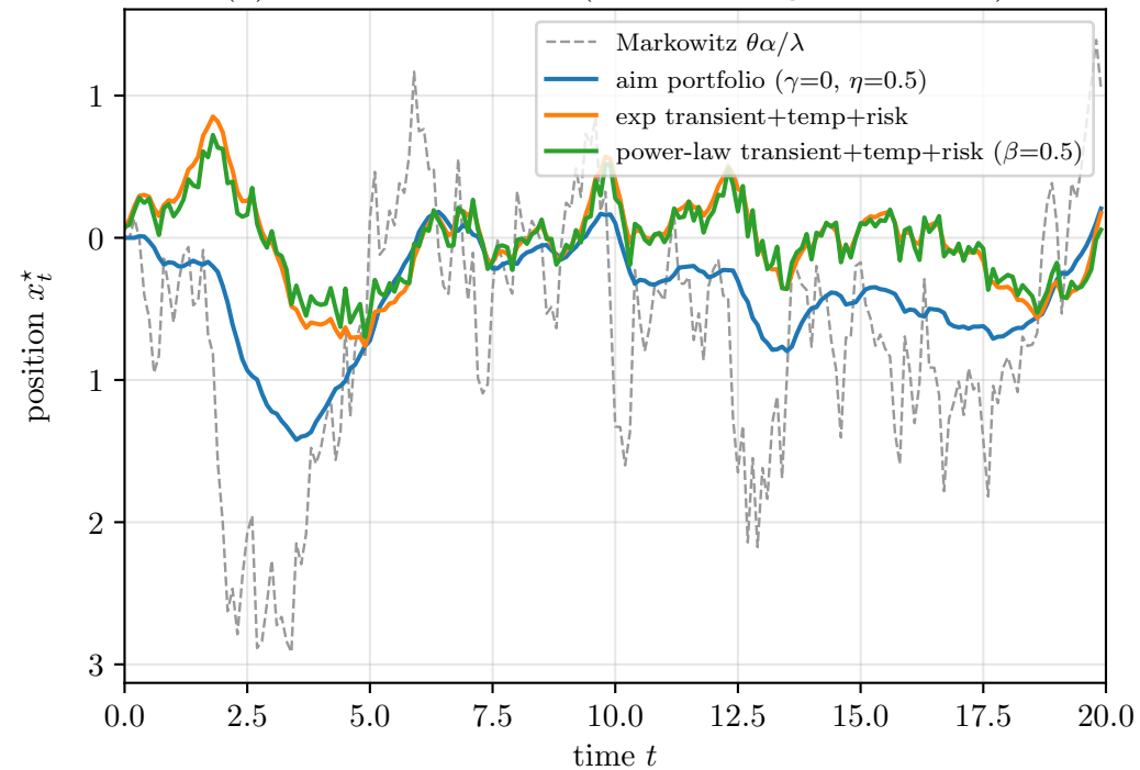
(a) optimal positions (same OU signal, \theta=\lambda=1 )
