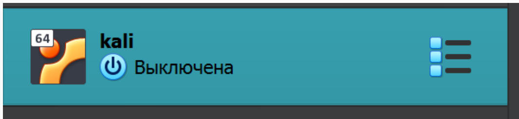
Рис. 3: Запуск VM
