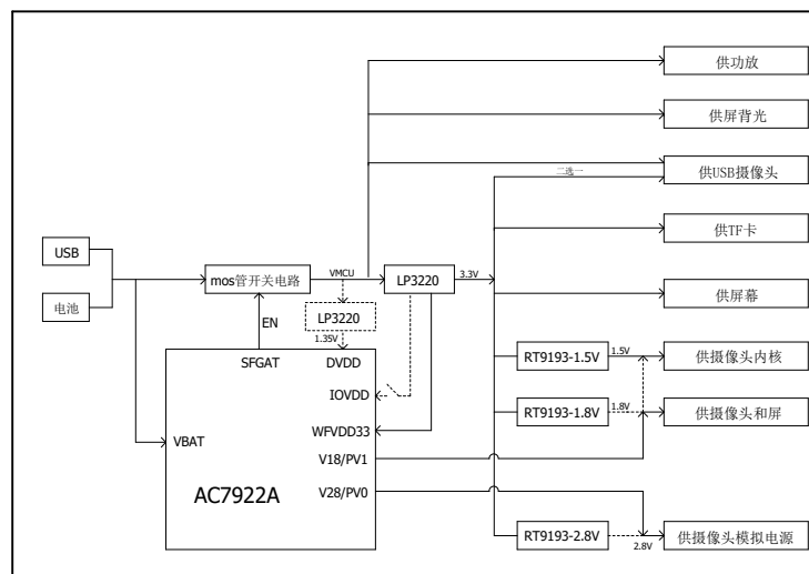
电源结构示意图
