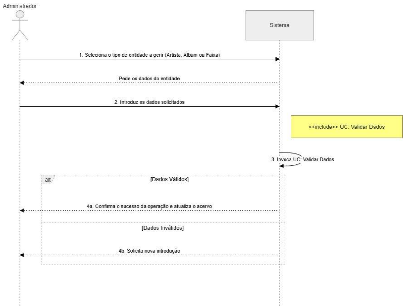
Figura 5 — Diagrama de Sequência: UC 1 — Gestão de Catálogo
