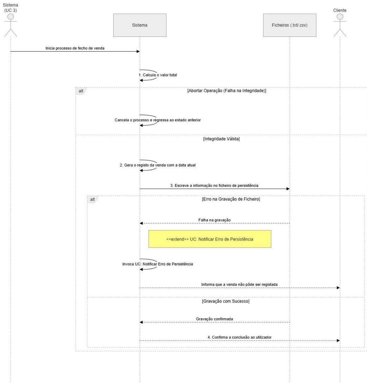
Figura 6 — Diagrama de Sequência: UC — Finalizar Transação
