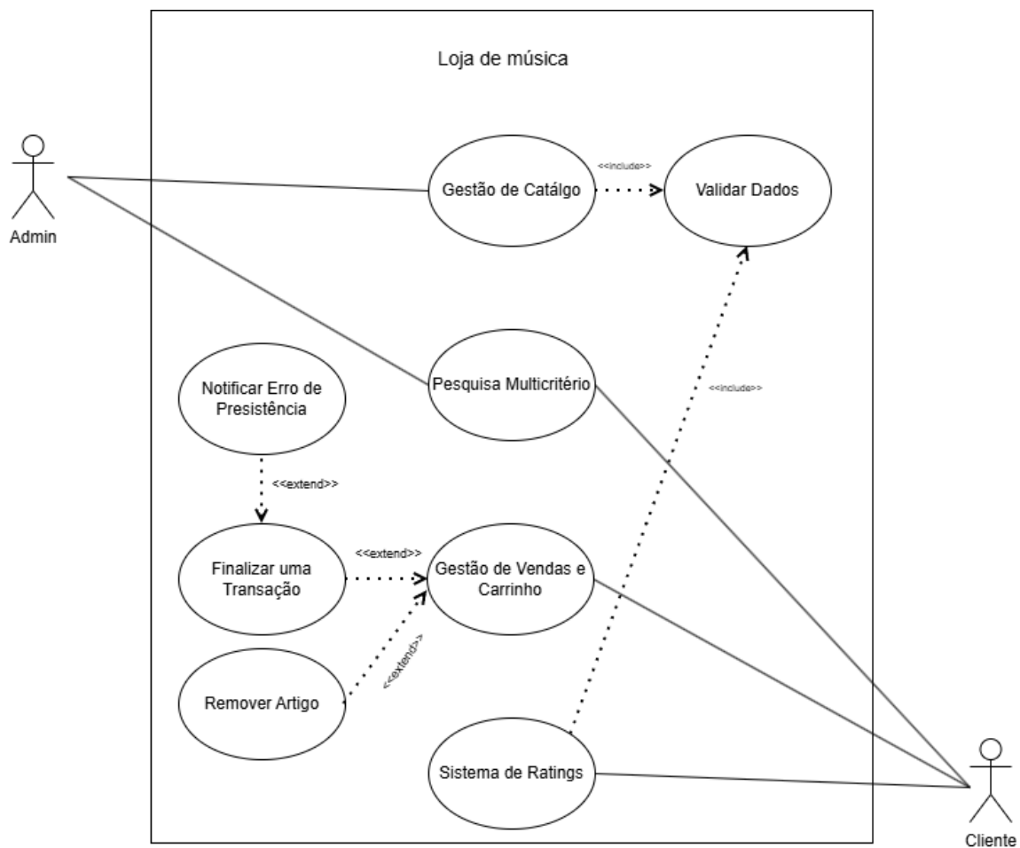
Figura 1 - Diagrama de Casos de Utilização da Loja de Música
