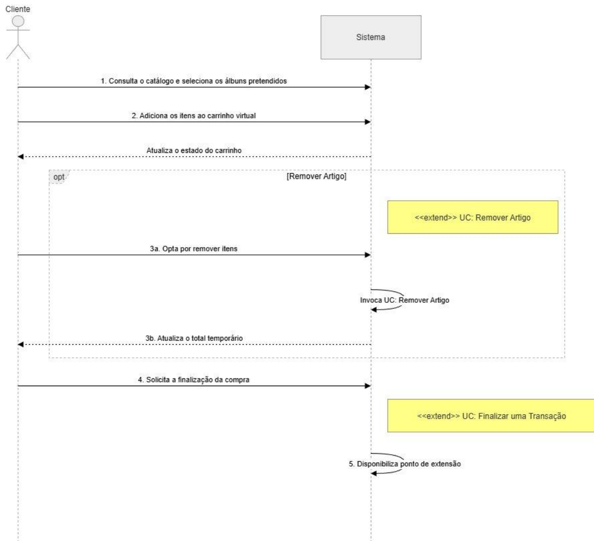
Figura 4 — Diagrama de Sequência: UC 3 — Gestão de Vendas e Carrinho
