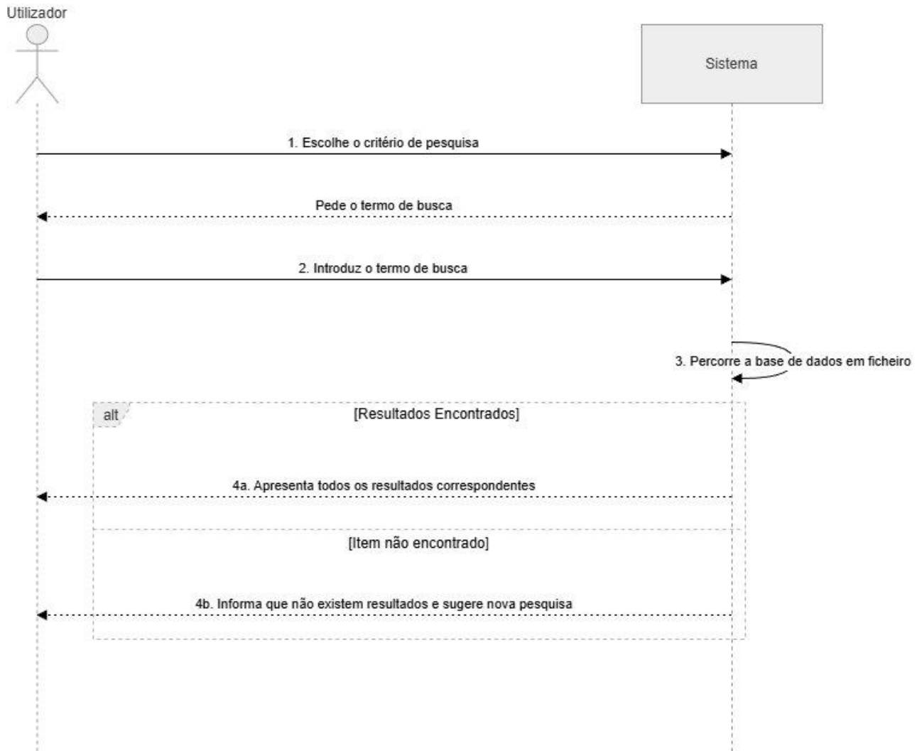
Figura 3 — Diagrama de Sequência: UC 2 — Pesquisa Multicritério
