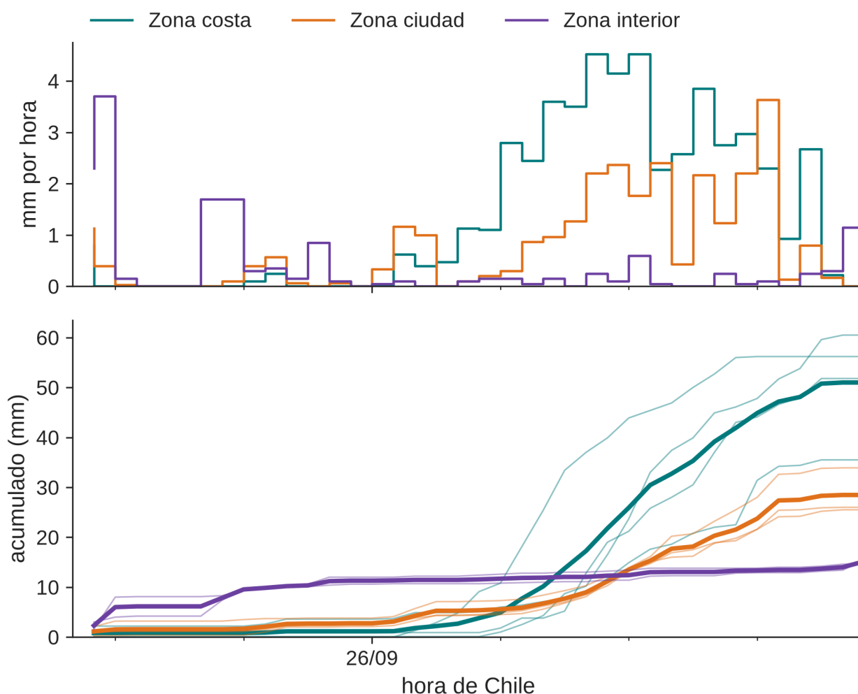
Figura 1. Arriba: lluvia horaria promedio de cada zona. Abajo: acumulado de la zona (línea gruesa) y de cada estación (líneas finas). Datos preliminares, sin control de calidad.
