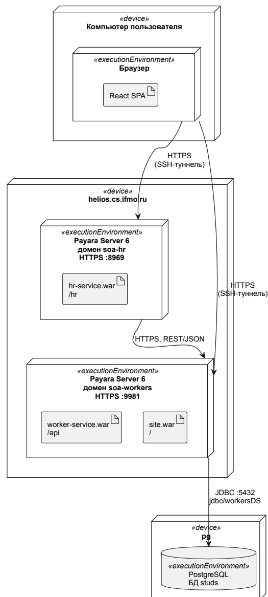
Рис. 1. Диаграмма развёртывания
