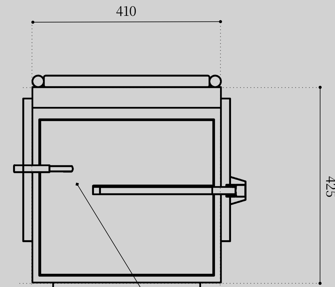
図4-1 1/5 平面図
