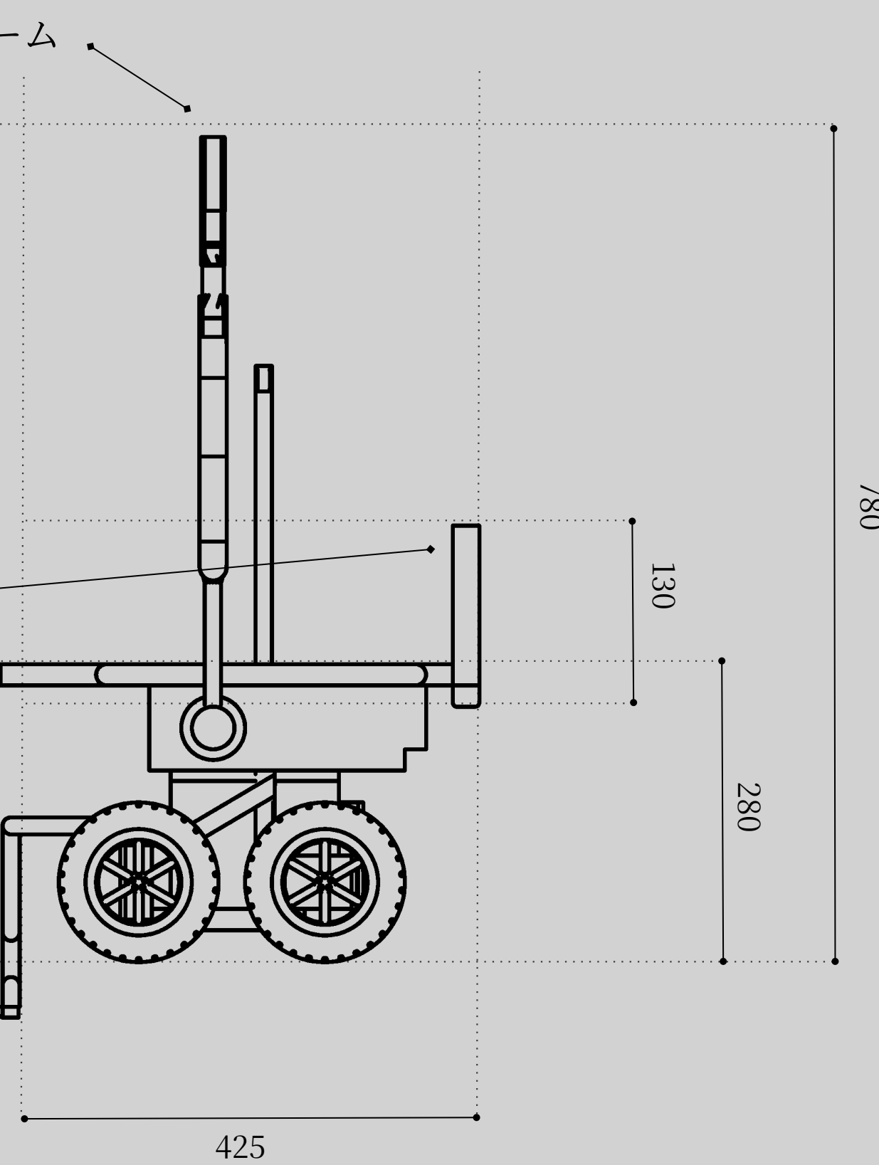
図4-3 1/5 右面立面図
