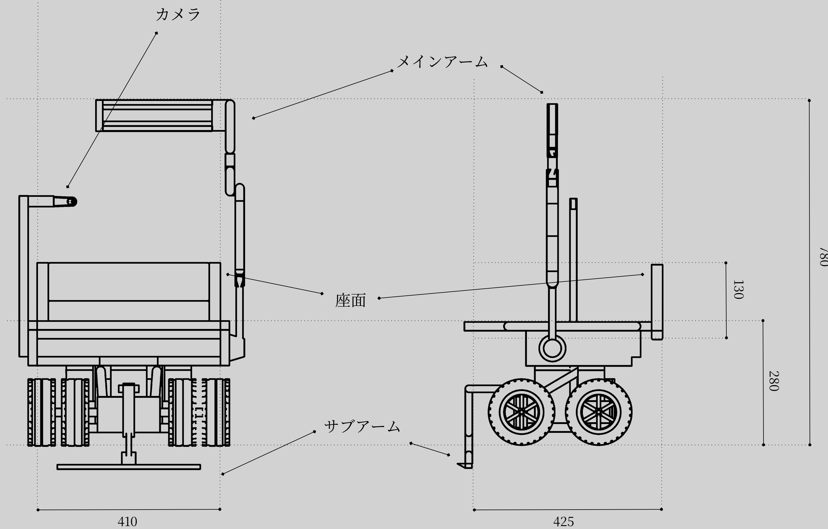
図4-2 1/5 前面立面図
