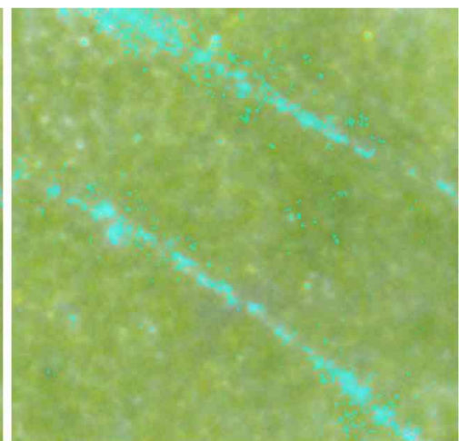
SmoothGrad
