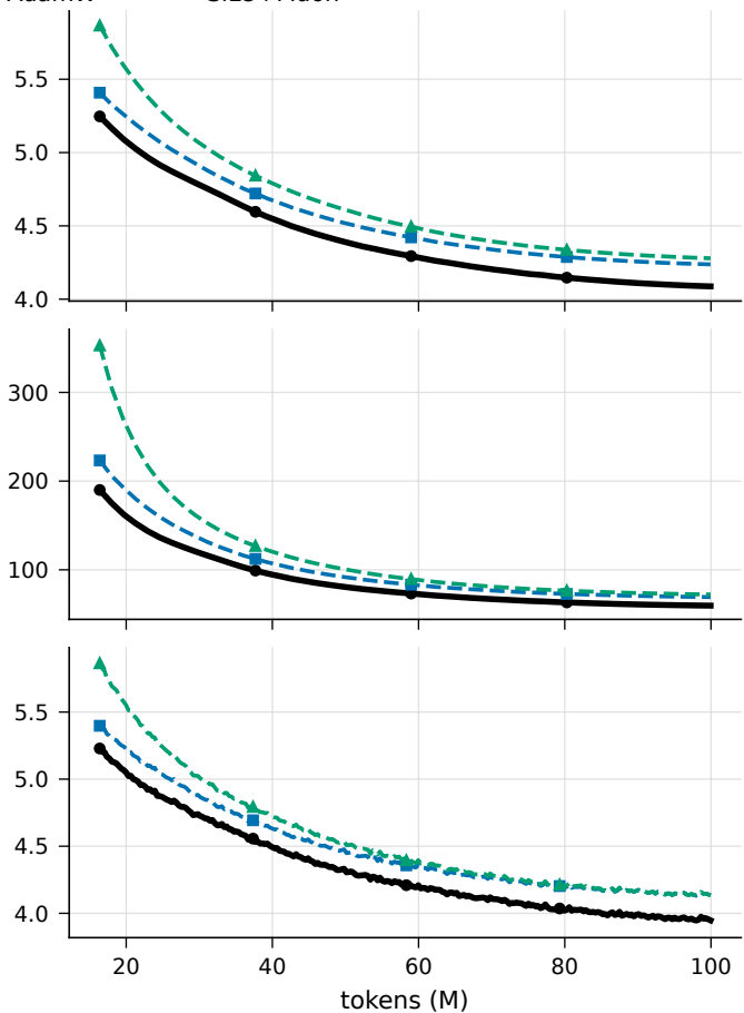
FineWeb-Edu
