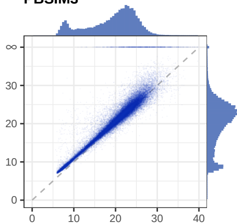
PBSIM3
