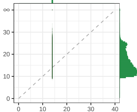
PBSIM3
