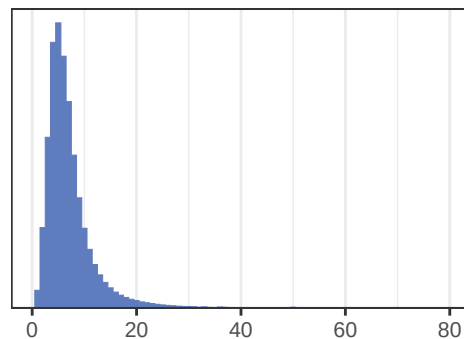
PBSIM3
