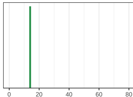
Irsim
