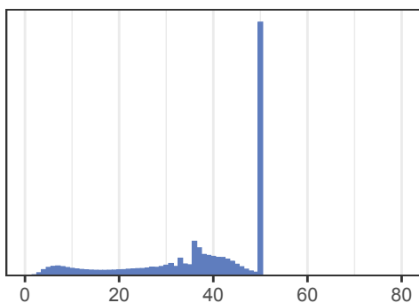
PBSIM3
