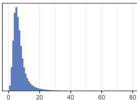
PBSIM3
