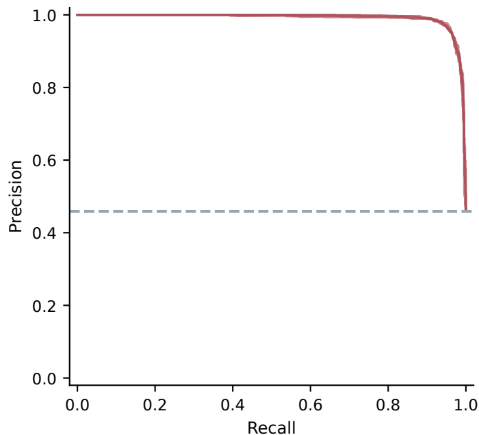
C Precision-recall · AUPRC 0.9912
