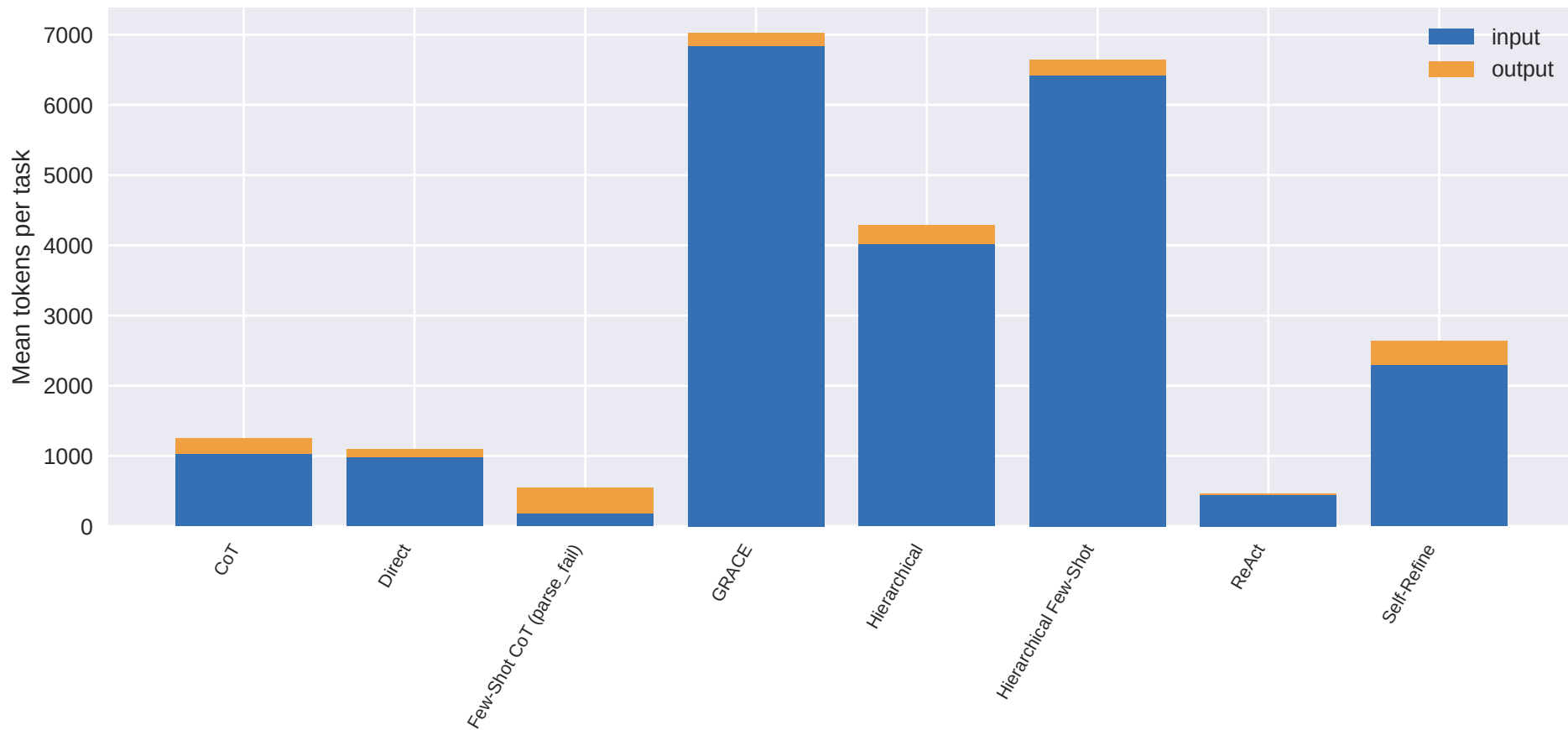
Token breakdown — model=mistral-nemo
