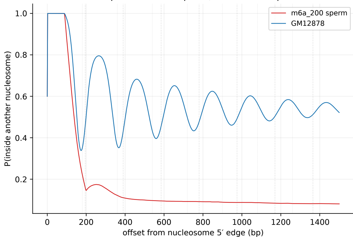
B. Zoom 0-1500 bp · dotted=180 bp NRL, dashed=195 bp NRL
