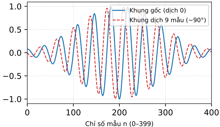
(a) Dạng sóng khung tại độ dịch 0 và 9 mẫu
