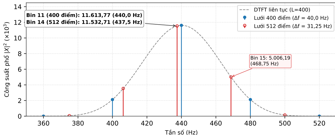
Hình 3: Đo lường thực nghiệm: Lưới 400 điểm (không đệm số 0, đỉnh trùng khít tại bin 11) so với Lưới 512 điểm (đệm 112 số 0, đỉnh tại bin 14 lệch 2,5 Hz sang 437,5 Hz). Đồ thị minh chứng rõ nét: đệm số 0 chỉ lấy mẫu dày hơn trên đường cong DTFT liên tục, không làm co hẹp búp chính vật lý của tín hiệu.
