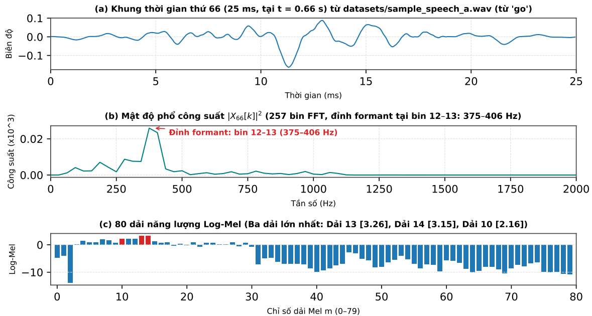
Hình 5: Đặc trưng phổ một khung tiếng nói thật trích xuất từ datasets/sample_speech_a.wav. (1) Bản chất: Ba tầng biểu diễn của khung âm thanh đỉnh (khung thứ 66, thời điểm t = 0,66 s) của từ phát âm “go” trong tập dữ liệu Speech Commands. (2) Điểm cần quan sát: Ở miền thời gian (a), dao động tuần hoàn thanh quản thể hiện rõ nét. Ở phổ công suất (b), năng lượng tập trung dày đặc ở các formant nguyên âm thấp tại bin 12–13 (375–406 Hz). Ở 80 thanh Log-Mel (c), ba dải năng lượng cực đại đo được chính xác là Dải 13 (382,1 Hz, giá trị 3,26 ), Dải 14 (416,3 Hz, giá trị 3,15 ), và Dải 10 (285,7 Hz, giá trị 2,16 ). (3) Ý nghĩa: Minh chứng tính toàn vẹn của đường truyền dữ liệu khi ánh xạ một nguyên âm thực tế thành vector đặc trưng 80 chiều cung cấp cho mô hình âm học.
