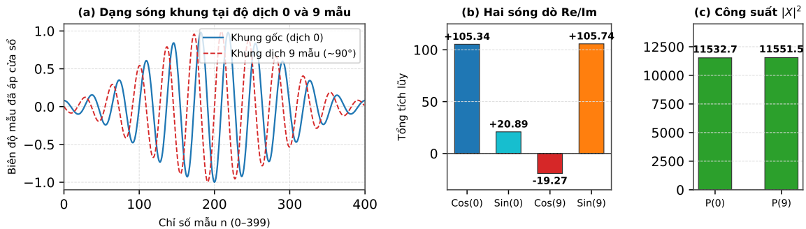
Hình 2: Đo lường thực nghiệm máy thu vuông pha trên tín hiệu kiểm chuẩn tổng hợp sample_tone440.wav . (a) Dạng sóng khung tại độ dịch 0 và 9 mẫu. (b) Hai sóng dò Re/Im: nhánh cosin sụt giảm sâu từ +105,34 về -19,27, nhánh sin vọt lên +105,74. (c) Công suất |X|^2 : tổng bình phương bất biến trước pha xuất hiện (11.532,71 \approx 11.551,50).
