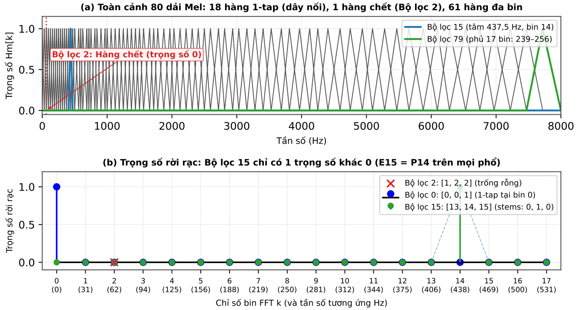
Hình 4: Hình học thực tế của Ngân hàng bộ lọc Mel trích xuất trực tiếp từ mã nguồn phòng thí nghiệm. (a) Toàn cảnh 80 dải Mel: nhận diện rõ Bộ lọc 2 là hàng chết (trọng số 0), 18 hàng 1-tap ở dải thấp, và các dải cao phủ rộng tới 17 bin. (b) Trọng số rời rạc: Bộ lọc 15 chỉ có đúng một trọng số khác 0 tại bin 14 ( E_{15} = P_{14} trên mọi phổ); đường tam giác nét đứt nhạt phía sau minh họa đường cong liên tục mà lưới FFT đã không thể lấy mẫu.
