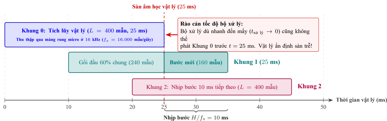
Hình 1.4a: Sàn trễ âm học so với tốc độ tính toán của bộ xử lý. (1) Nó là gì: Trục thời gian luồng âm thanh dòng thể hiện quá trình tích lũy khung vật lý và nhịp phát định kỳ của các bước nhảy. (2) Nhìn vào đâu: Khung 0 bắt buộc phải tích lũy đủ 25 ms (400 mẫu) áp suất âm học trước khi có thể bắt đầu xử lý; bộ xử lý lý thuyết dù có thời gian thực thi tiệm cận 0 cũng không thể vượt qua sàn vật lý này. Các khung kế tiếp tịnh tiến mỗi 10 ms (160 mẫu) với vùng gối đầu 60% (240 mẫu). (3) Nó chứng minh điều gì: Độ trễ thời gian thực trong hệ thống âm thanh biên bị chi phối nghiêm ngặt bởi quy luật truyền sóng và kích thước cửa sổ, không phụ thuộc vào tần số xung nhịp bộ xử lý.
