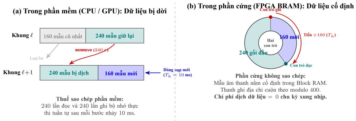
Hình 1.2a: Sự đối lập cơ học giữa thao tác dịch bộ nhớ trong phần mềm (a) và cơ chế bộ đệm vòng phần cứng (b) cho khung 400 mẫu với bước nhảy 160 mẫu ( T_h = 10 ms). Trong khi phần mềm phải liên tục đọc và ghi 240 mẫu qua bus sau mỗi bước nhảy, phần cứng giữ cố định dữ liệu trong Block RAM và chỉ dịch chuyển hai thanh ghi con trỏ theo modulo 400, triệt tiêu hoàn toàn chi phí dịch chuyển mẫu.
