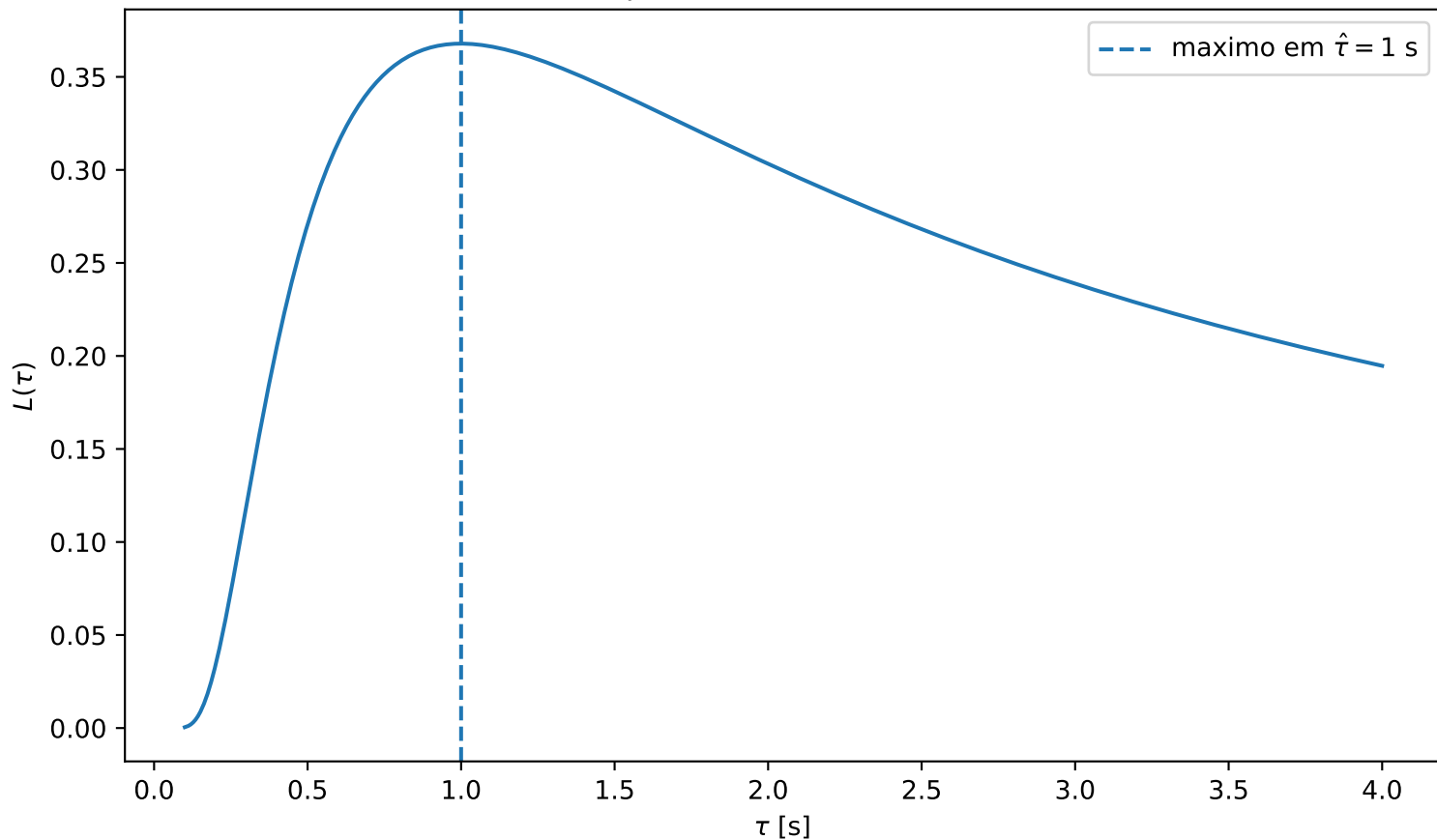
Likelihood para uma unica medida t = 1 s
