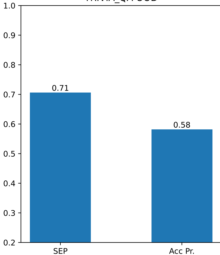
TRIVIA_QA OOD
