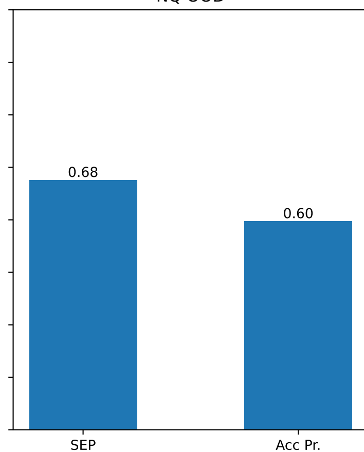
NQ OOD
