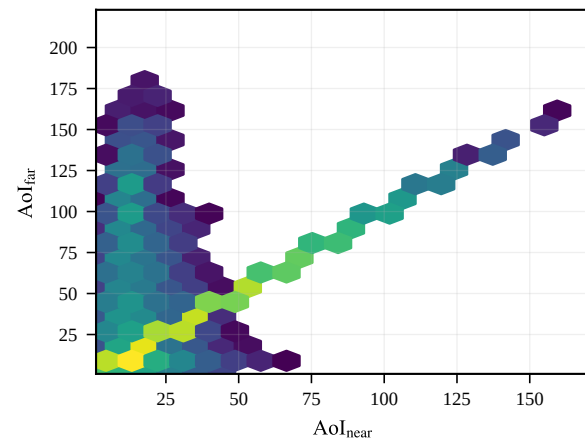
Action a=5
