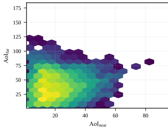
Action a=7
