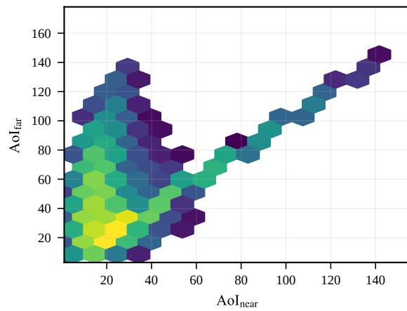
Action a=4
