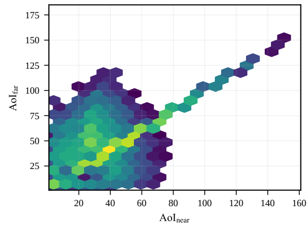
Action a=5
