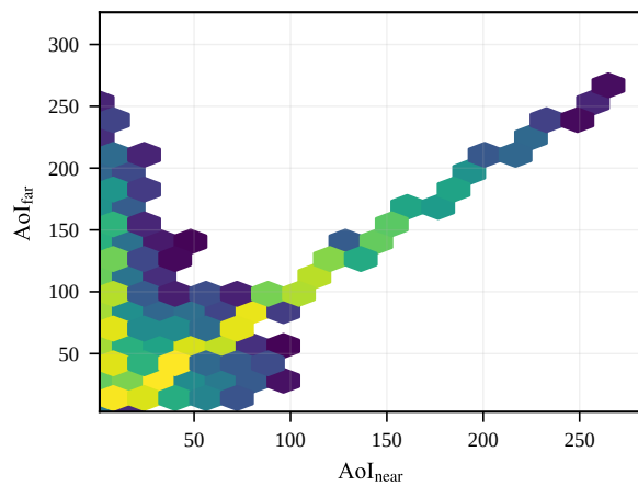
Action a=7
