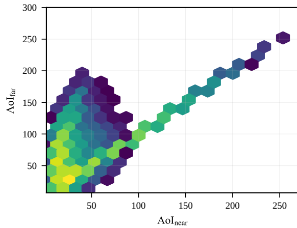
Action a=4
