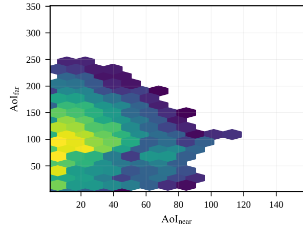
Action a=6
