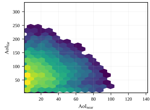
Action a=3
