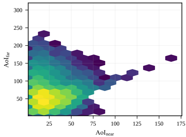
Action a=7
