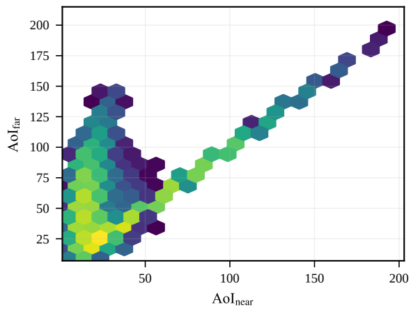
Action a=4
