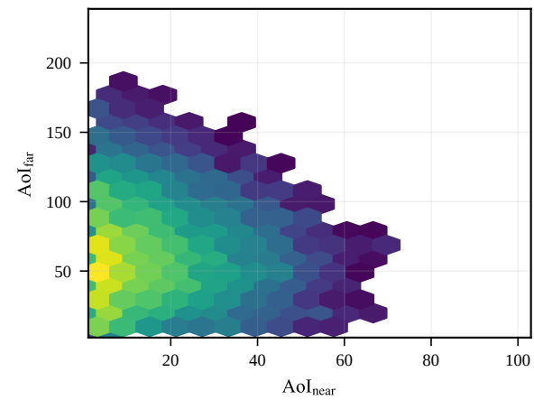
Action a=3
