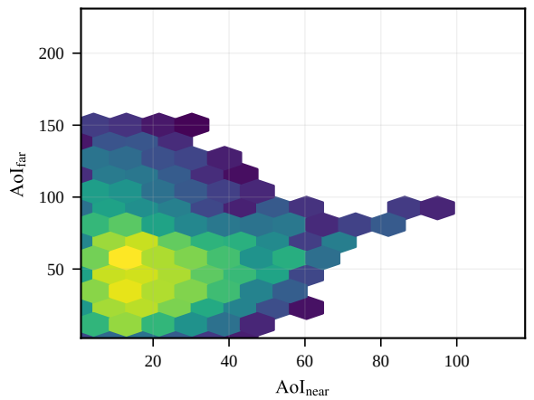
Action a=7
