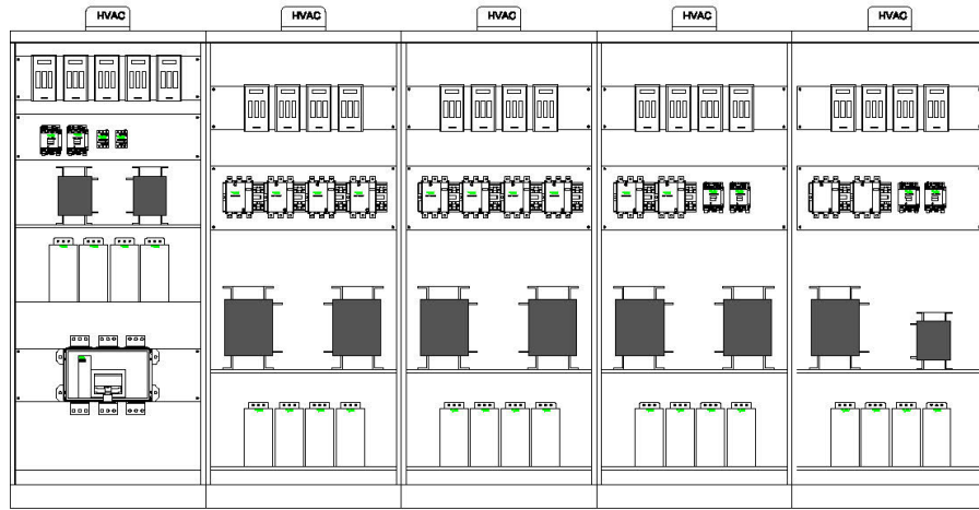
PANO İÇ GÖRÜNÜŞ
