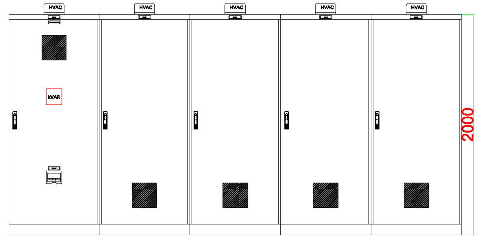
PANO ÖN GÖRÜNÜŞ
