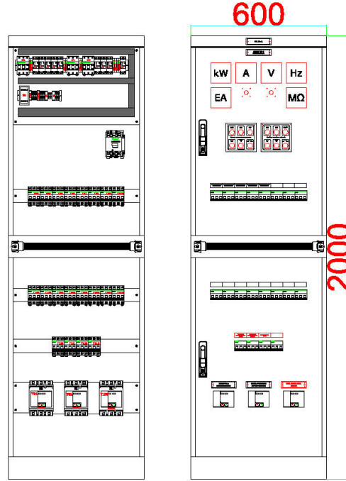
PANO İÇ VE ÖN GÖRÜNÜŞ
