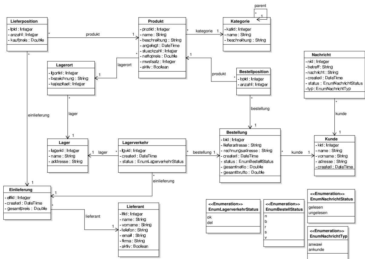
Abbildung 1.1: Spezifikation der Daten des Warenwirtschaftssystems als Klassendiagramm
