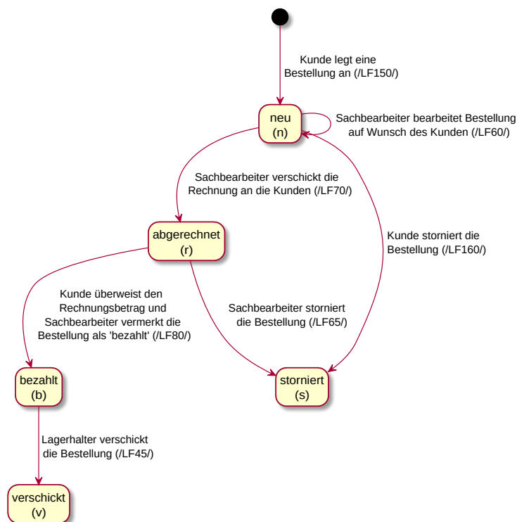
Abbildung 2.1: Zustandsdiagramm einer Bestellung im WAWI
