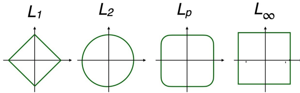
Figura 13.1: Familia de normas L_p Fuente: Dr Will Wood
