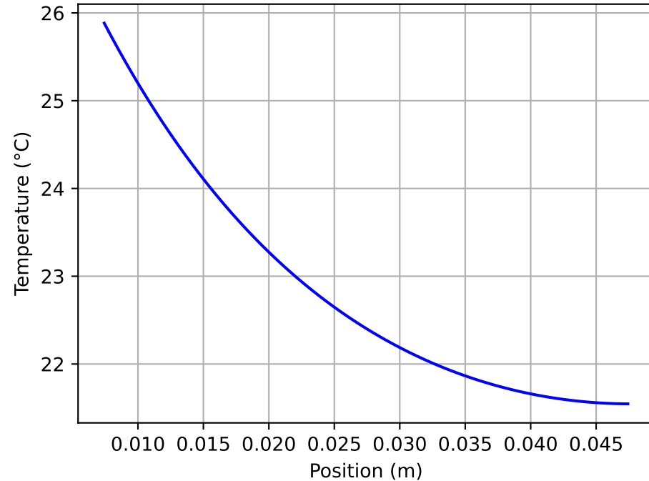
Fin Temperature
