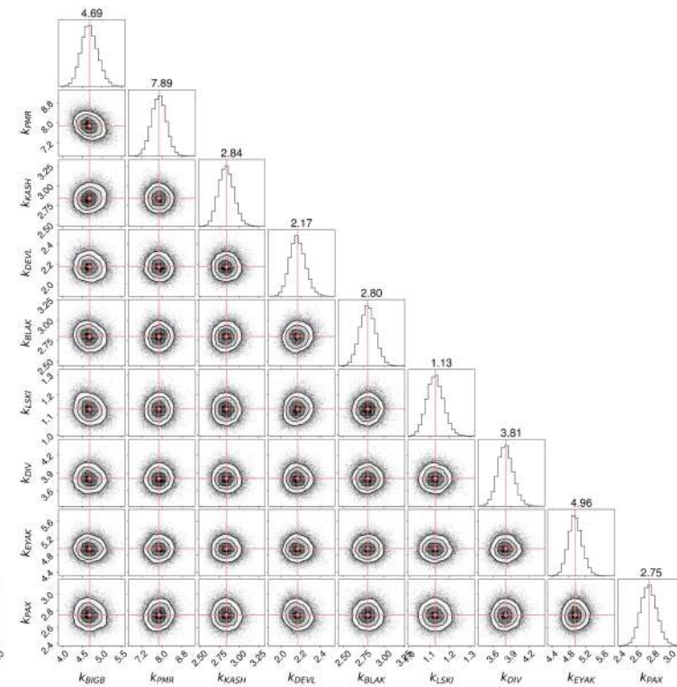
c) Posterior of noise parameters (correlated noise)
