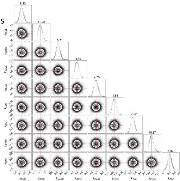
b) Posterior of noise parameters (uncorrelated noise)
