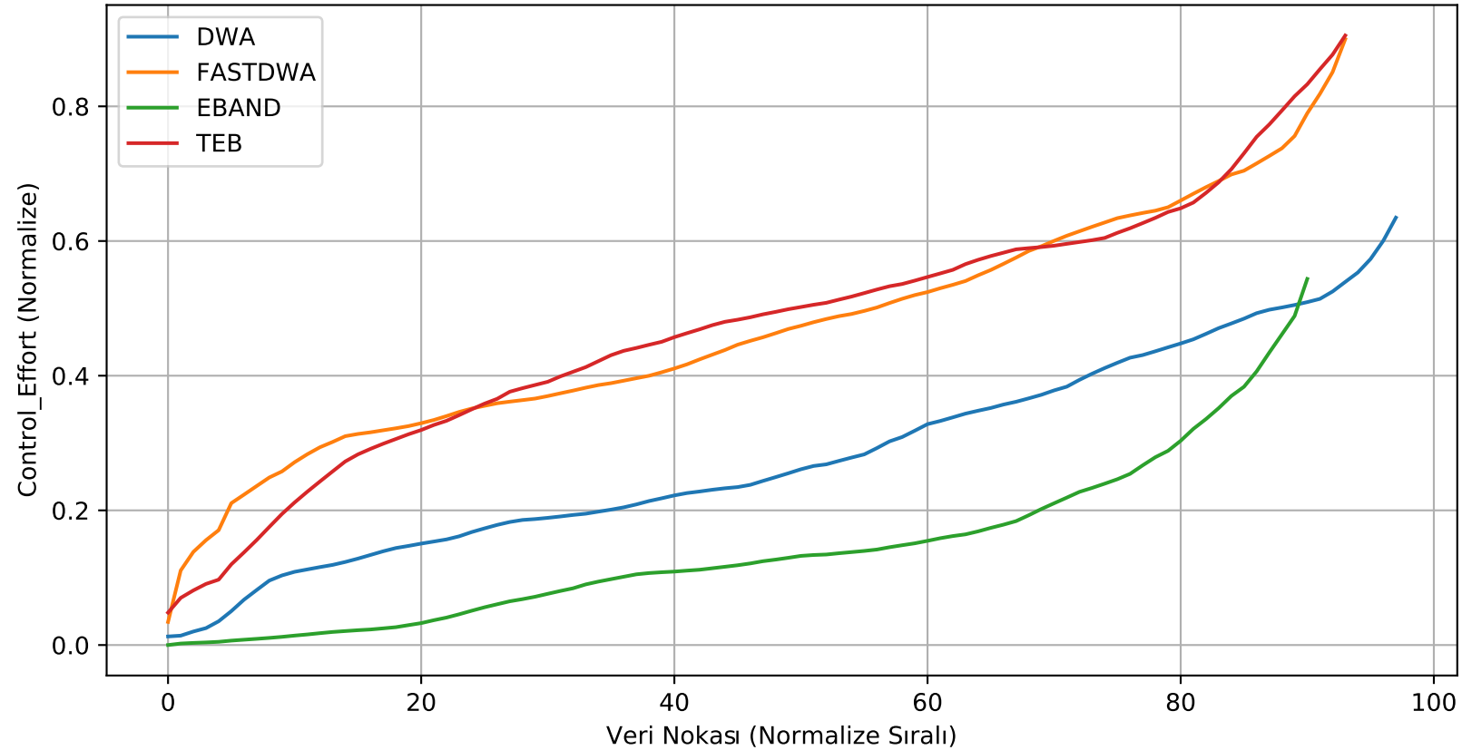
Control_Effort - Karşılaştırmalı (Normalize + Smooth)
