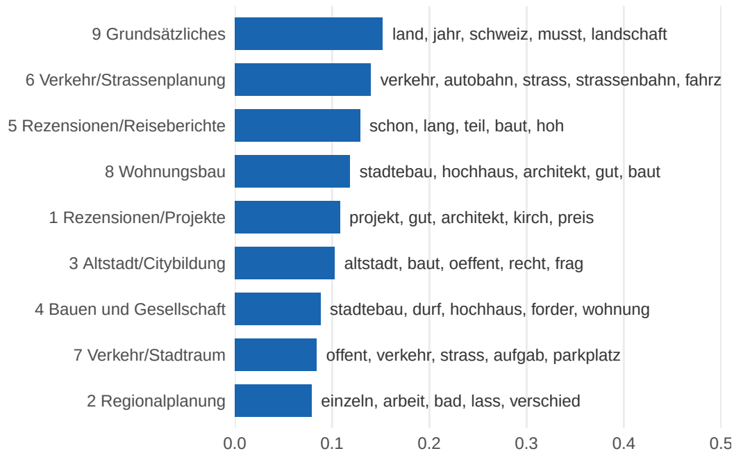
Abbildung 18: Topics im Modell mit Covariates (publication + pol_mandat + fachpublikum) mit dargestellten Proportionen und je fünf charakteristischen features
