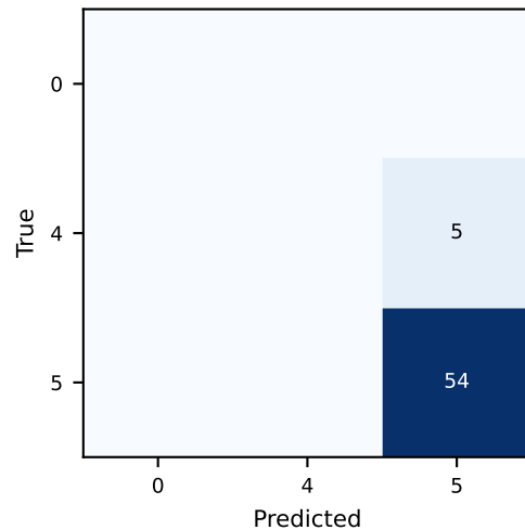
Star (ViT-S)
