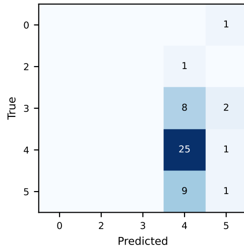
Star (ViT-S)
