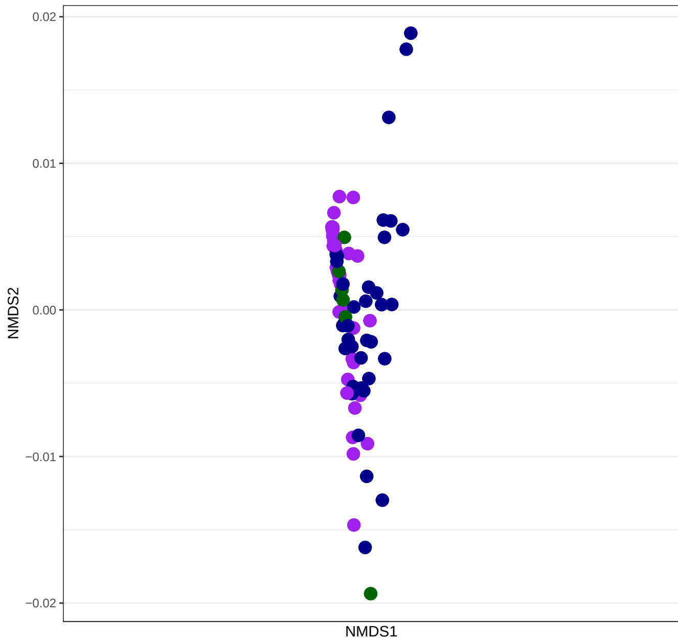
Pielou NMDS
