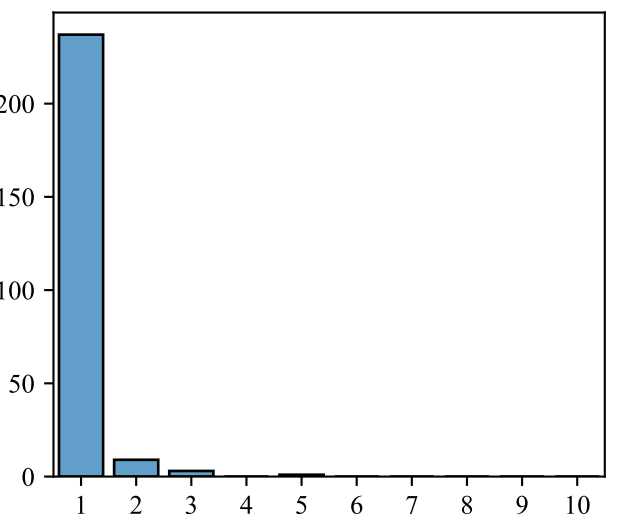
gemma-3-27b
