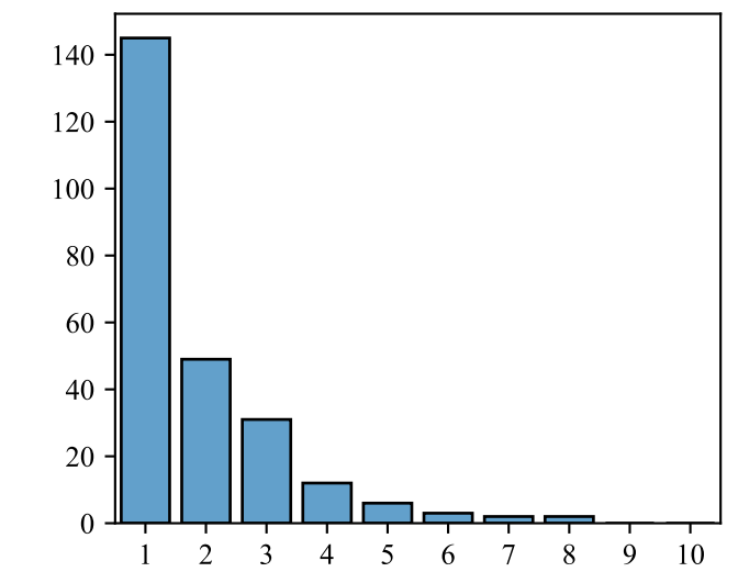
Mistral-Nemo-7B
