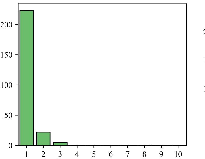
DeepSeek-Qwen-32B
