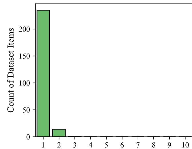
SVamp
