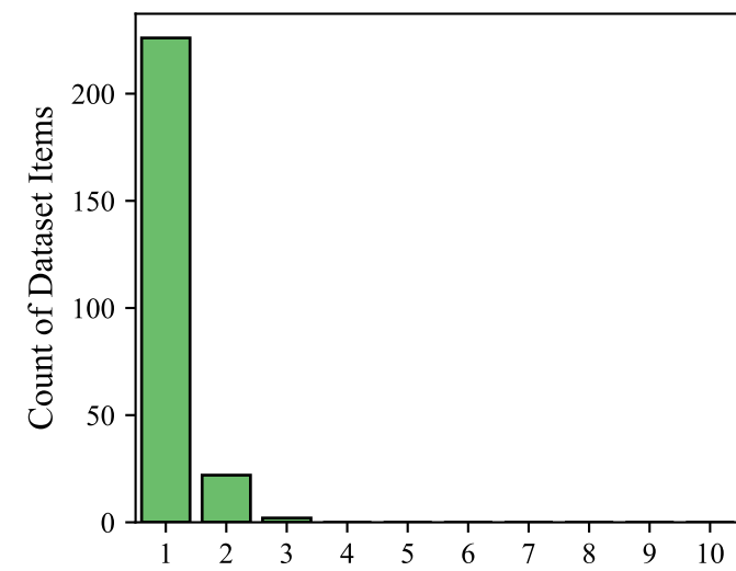
gpt-oss-20b
