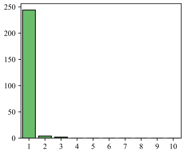
Qwen3-30B-A3B-Thinking
