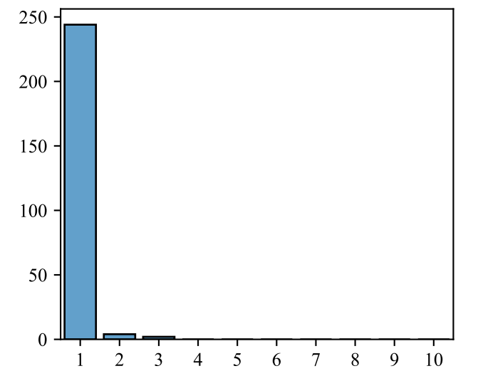
Llama-4-Scout-17B
