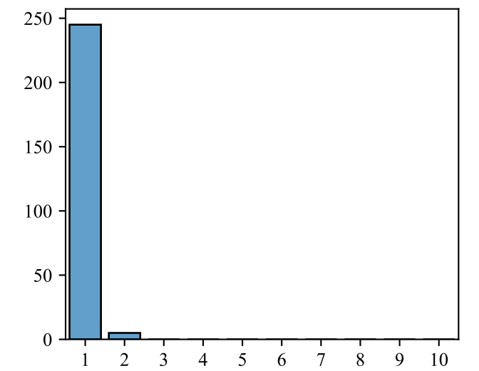
Llama-3.3-70B
