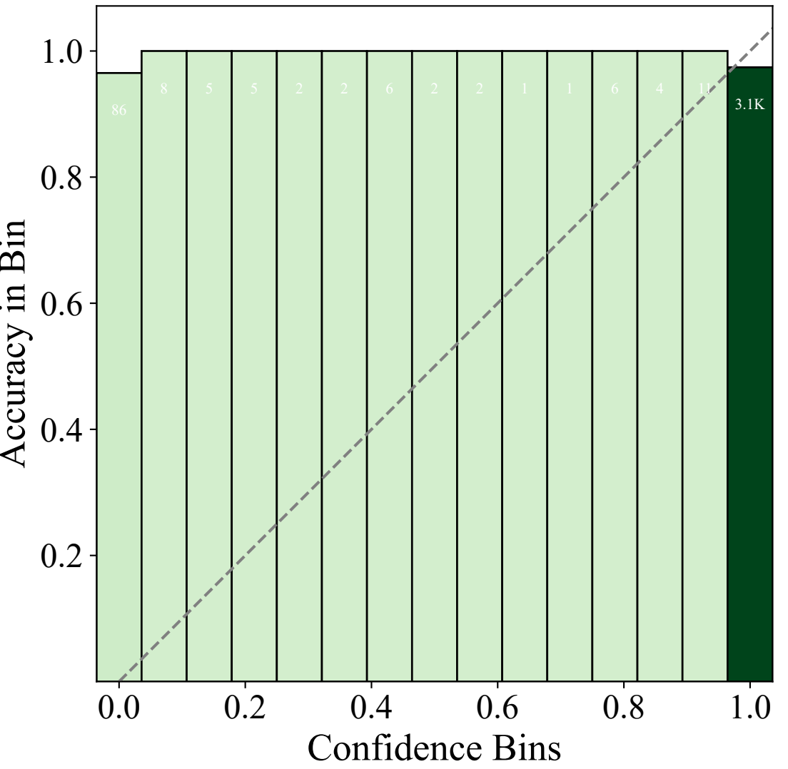
P(True)
