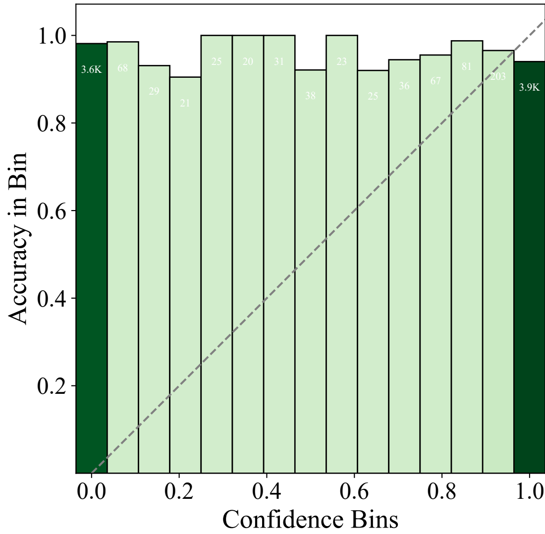
P(True)
