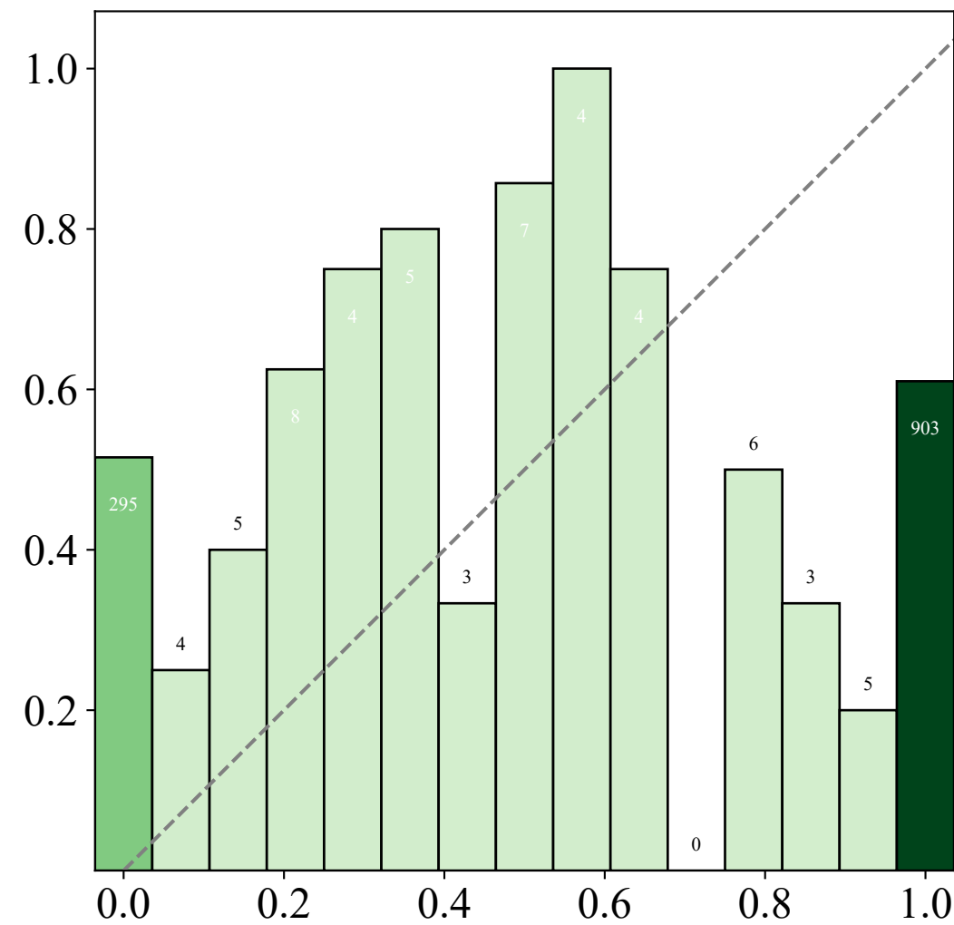
P(True)
