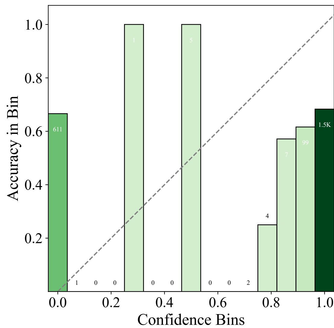
GSM8K
