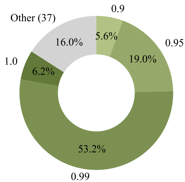
gpt-oss-20b
