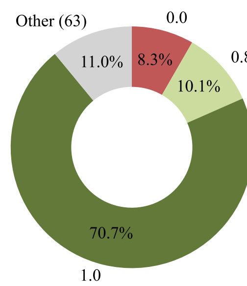
Llama-4-Scout-17B
