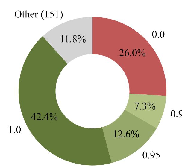
DeepSeek-Qwen-32B
