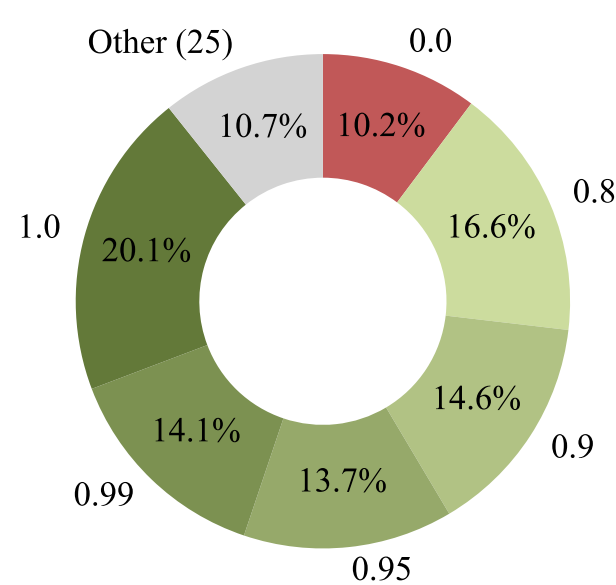
Llama-3.3-70B
