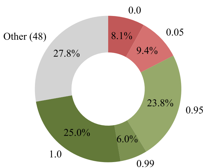
google/gemma-3-27b
