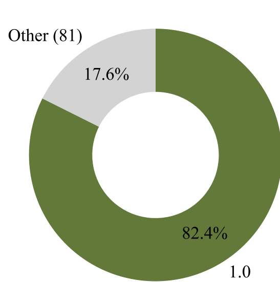
Qwen3-30B-A3B-Thinking
