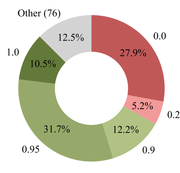
Mistral-Nemo-7B
